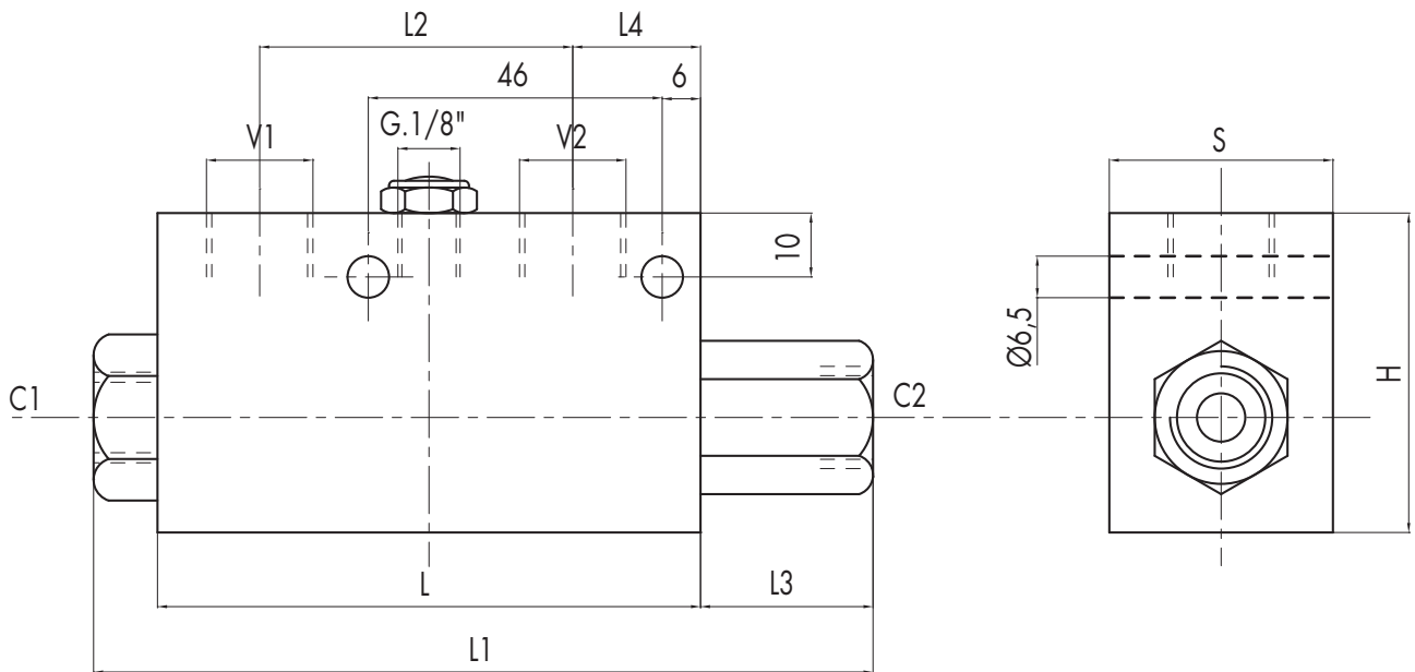
SCHEMA DI MONTAGGIO MOUNTING DIAGRAM
